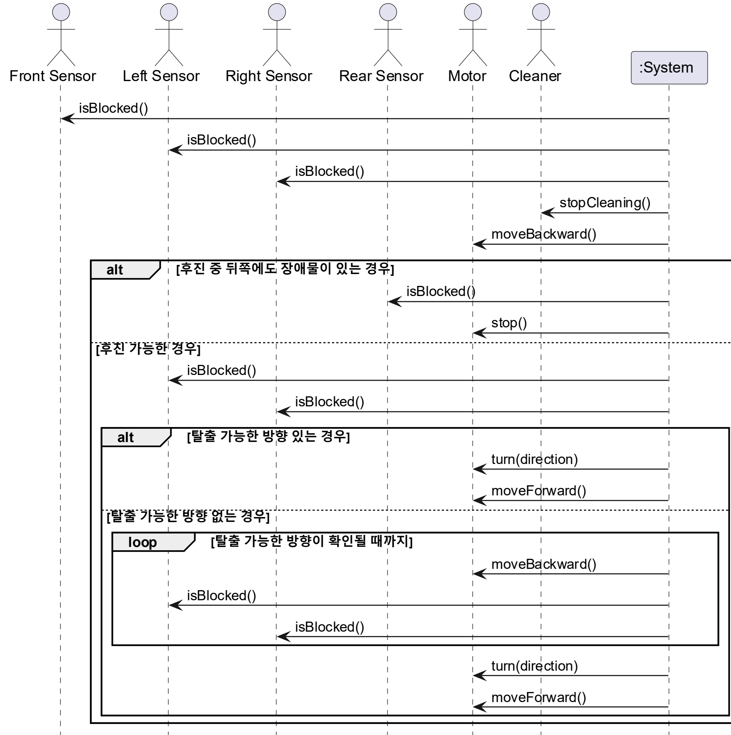
UC-04 모든 방향 막혔을 때 탈출 - SSD
