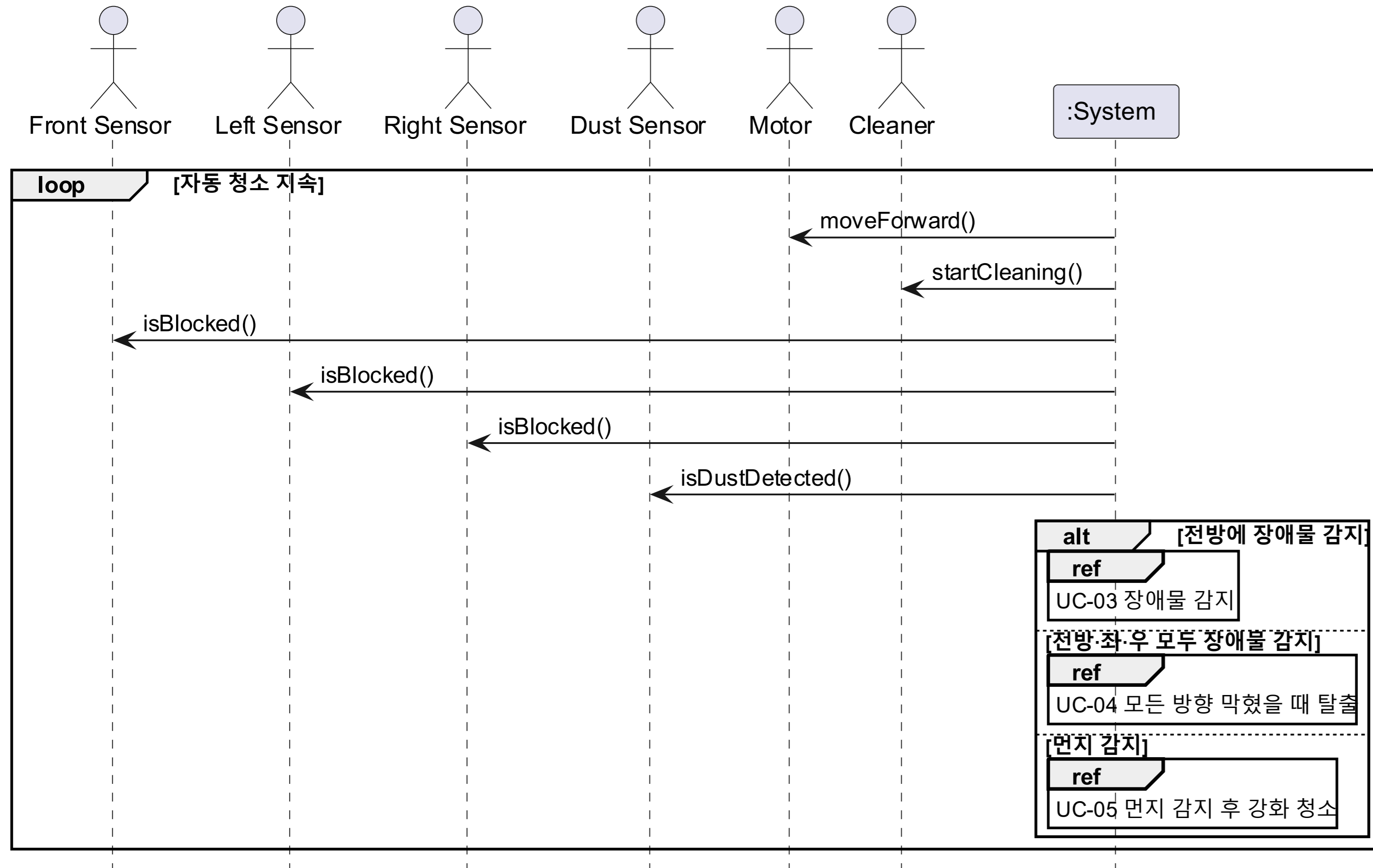
UC-02 자동 청소 수행 - SSD
