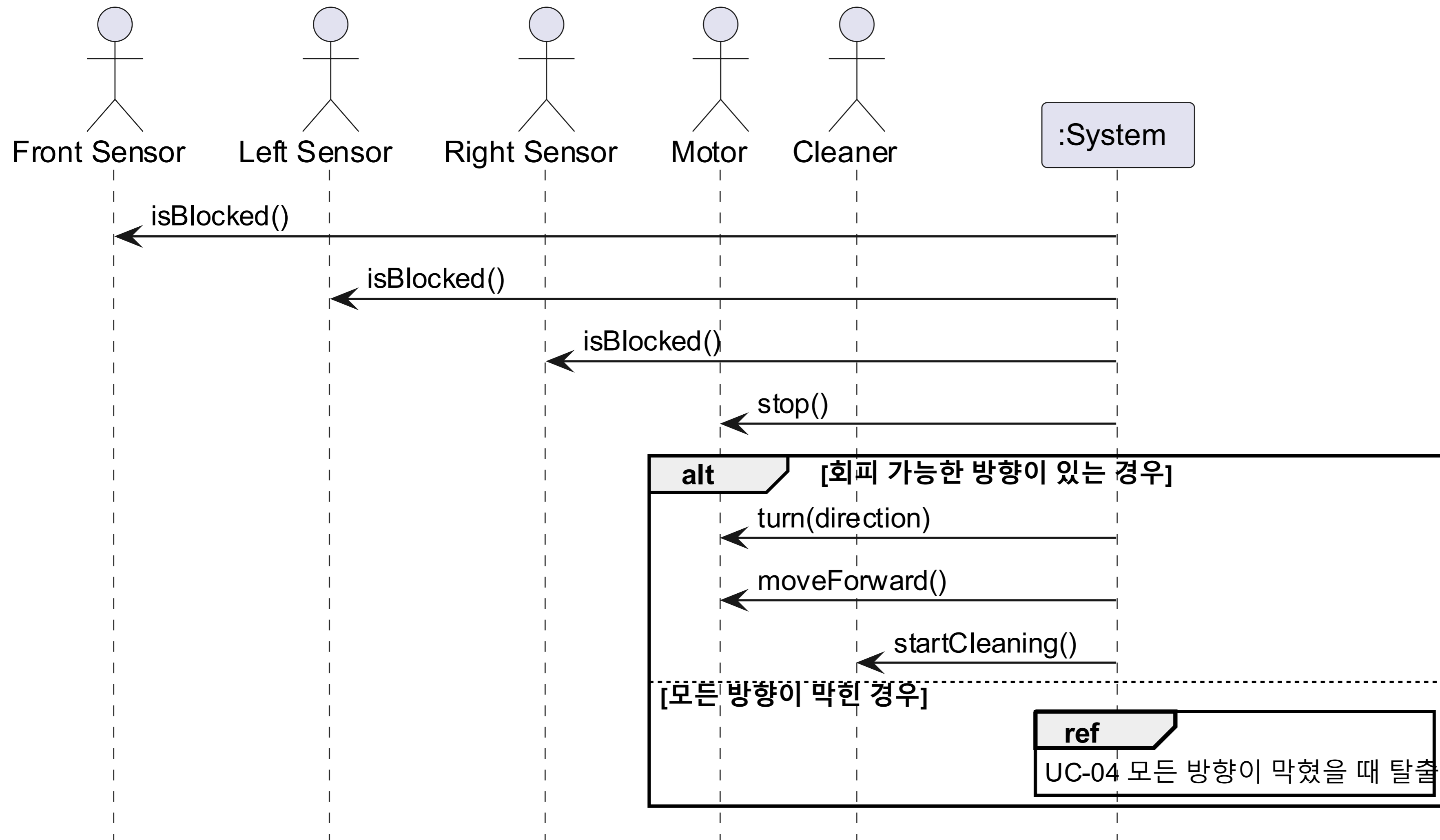
UC-03 장애물 감지 - SSD
